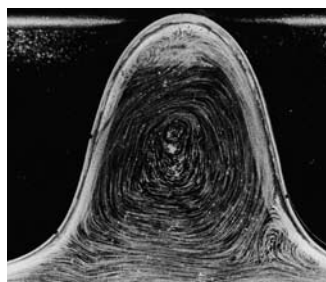
Gewellte Bauform: Maximale Wärmeübertragung/Durchströmung bis in die Randbereiche.
