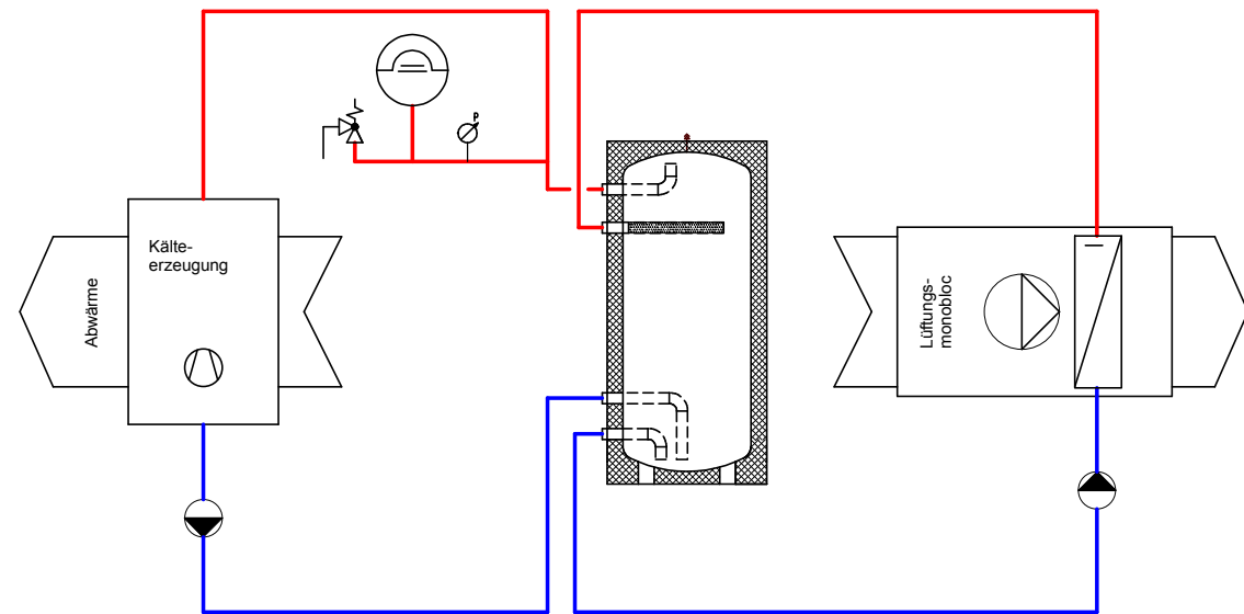
Prinzipschema Kälte
