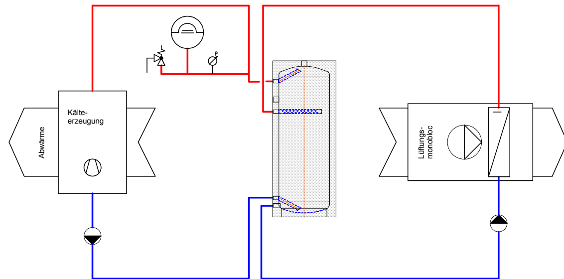
Prinzipschema Kälte
