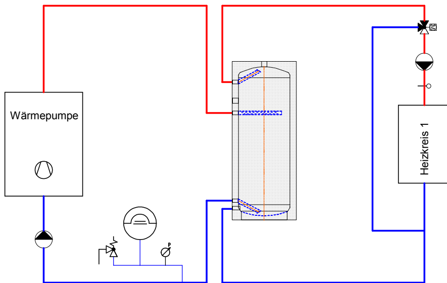
Prinzipschema Heizung
