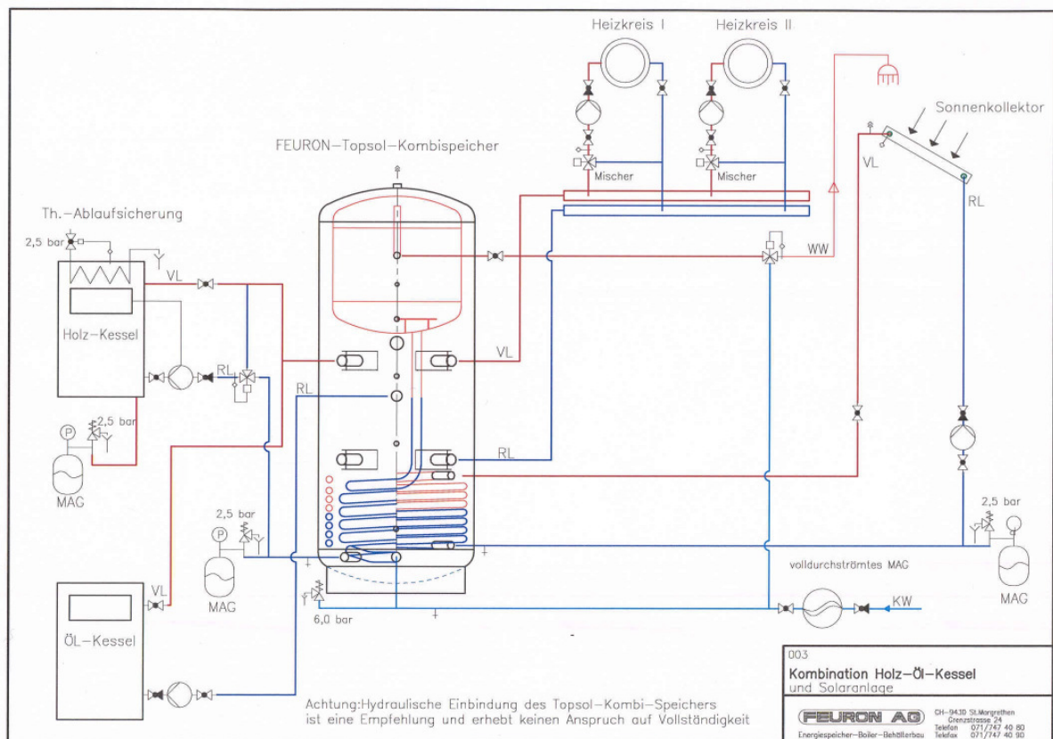
Abb. 3 Hydraulik Schema
