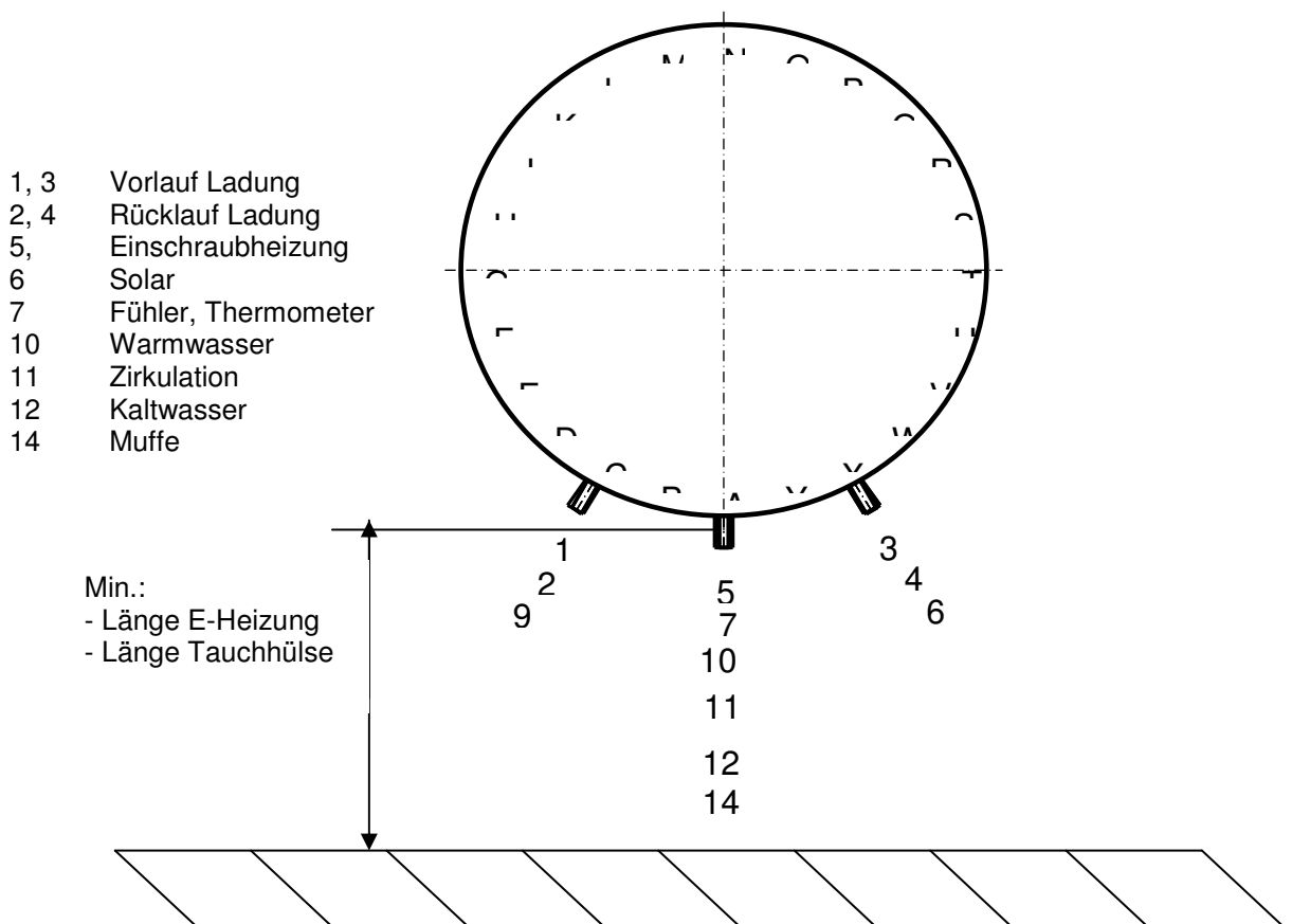
Abb. 1 Speicheraufstellung im Installationsraum
